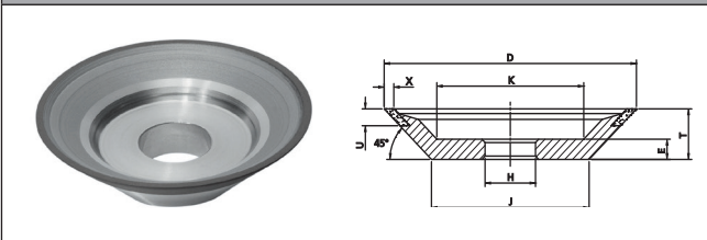
Form 12A2 45°
