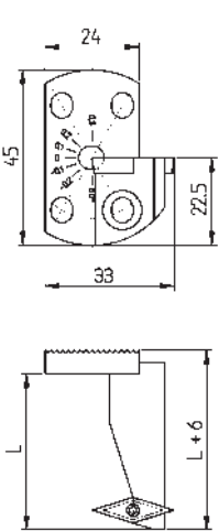
SVNCR11 (Ausführung rechts) (Version right)
