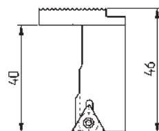
Ausführung rechts Version right
