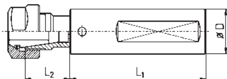
Beispiel - example: Halter GFU mit abgesetzter Spannfläche FL Holder GFU with enclosed clamping flat FL
