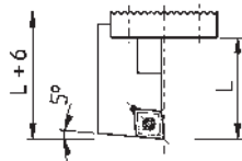
SCLCL06 (Ausführung links) (Version left)
