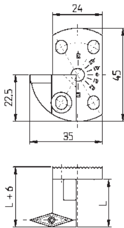
HVWPA-SVNCR11 (Ausführung rechts außen) (Version right external)
