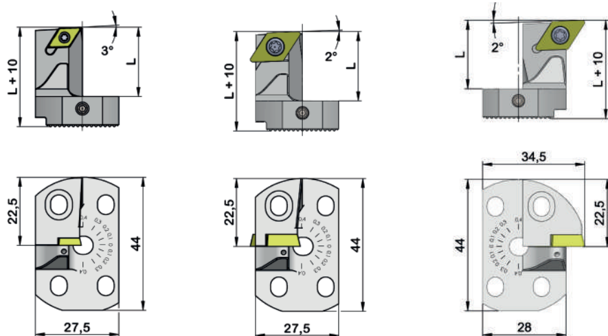
HVWPAX-SDJCR11 (Ausführung rechts außen) (Version right external)
