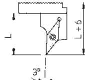
SVUCR11 (Ausführung rechts) (Version right)
