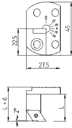
SDJCL11 (Ausführung links) (Version left)
