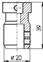
Bild 1: Halter - holder
