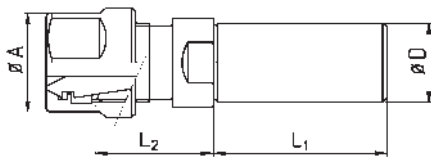
Beisp. - expl.: Mutter - nut UM/ER16
