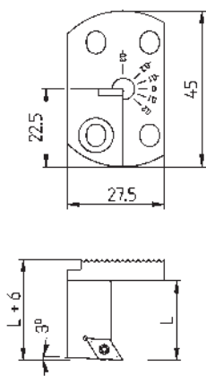
SDJCL07 (Ausführung links) (Version left)
