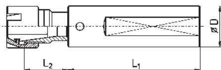
Beispiel - example: Halter GFM mit durchgehender Spannfläche WD Holder GFM with clamping flat throughout WD
