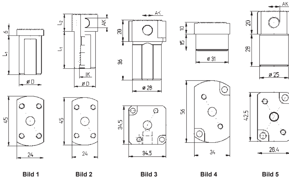
Standardschaft mit innerer Kühlmittelfuhr (AK / IK) Standard shank with inner coolant (AK / IK)
